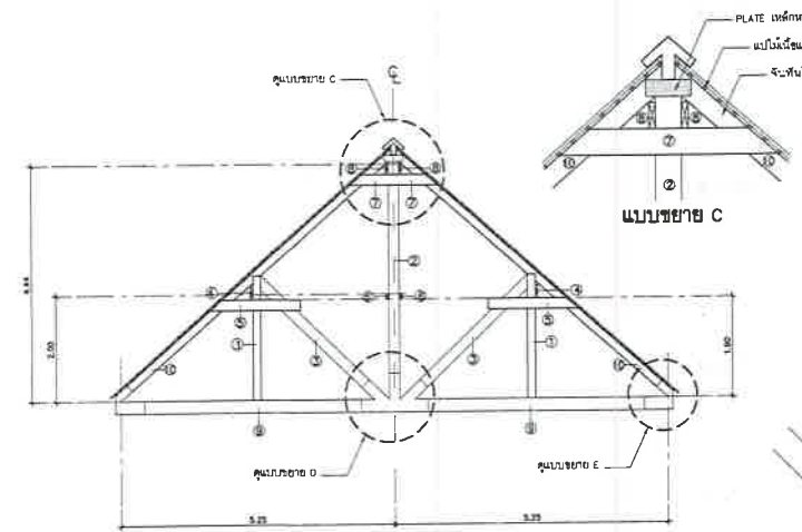
รูปตัด B-B (เดิม) ขนาดจริง 1:30
