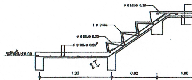
แบบขยายบันได มาตราส่วน
