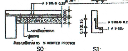
แบบขยายพื้น มาตราส่วน 1:25
