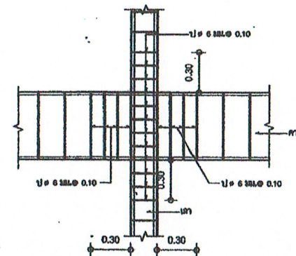
แผนผังการเสริมเหล็กปอดกิโลเมตรรอยต่อและคานทั่วไป
