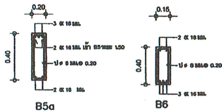
แบบขยายคาน มาตราส่วน 1:25
