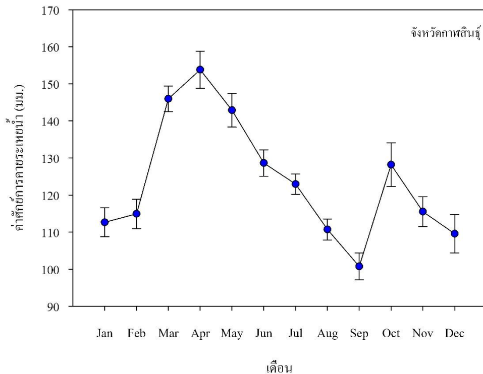
ภาพที่ ๓ กราฟแสดงค่าเฉลี่ยการคายระเหยน้ำ (มม.) ในแต่ละเดือนของจังหวัดกาฬสินธุ์ (ค่าเฉลี่ย ๑๐ ปี พ.ศ. ๒๕๔๒-๒๕๕๑, แหล่งข้อมูล: กรมอุตุนิยมวิทยา)
