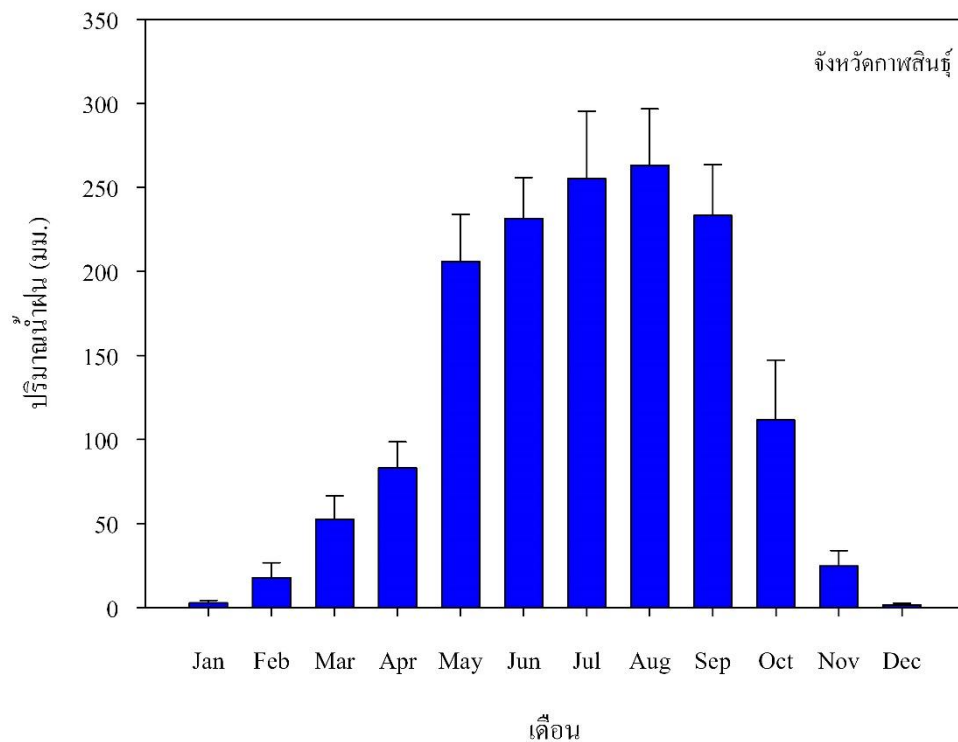
ภาพที่ ๔ กราฟแสดงปริมาณน้ำฝนสะสมในแต่ละเดือนของจังหวัดกาฬสินธุ์ (ค่าเฉลี่ย ๑๐ ปี ๒๕๔๒-๒๕๕๑, แหล่งข้อมูล: กรมอุตุนิยมวิทยา)
