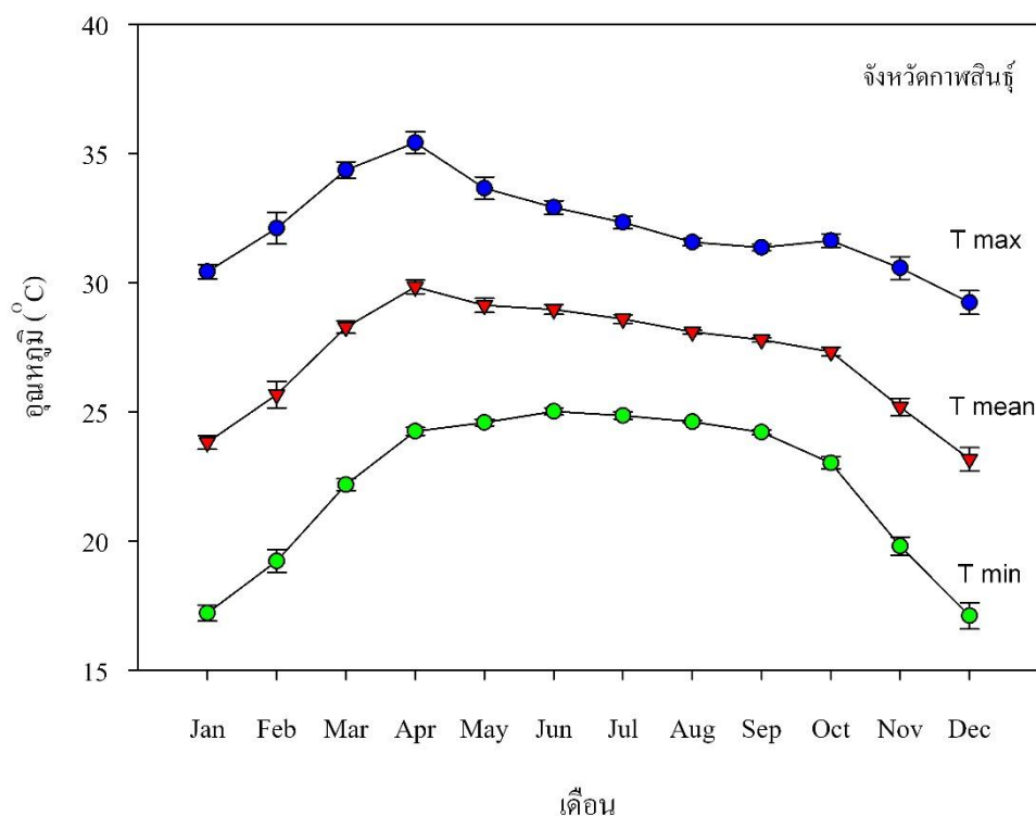
ภาพที่ ๑ กราฟแสดงอุณหภูมิในแต่ละเดือนของจังหวัดกาฬสินธุ์ ประกอบด้วย อุณหภูมิสูงสุด (T max) ต่ำสุด (T min ) เฉลี่ย (T mean) (ค่าเฉลี่ย ๑๐ ปี, พ.ศ. ๒๕๔๒-๒๕๕๑ แหล่งข้อมูล: กรมอุตุนิยมวิทยา)
