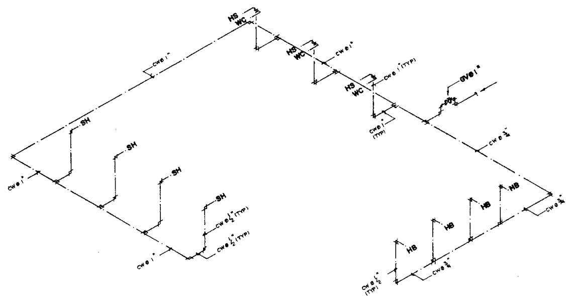
ISOMETRIC DIAGRAM OF COLD WATER SUPPLY PIPE สำหรับห้องน้ำหญิง NOT TO SCALE
