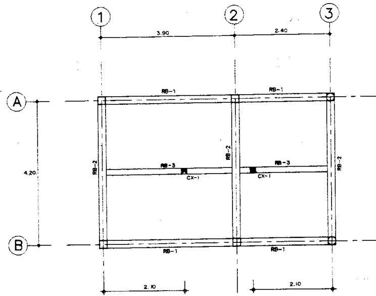
แปลนโครงสร้างระดับอะไหล่ ขนาดส่วน 1 : 50
