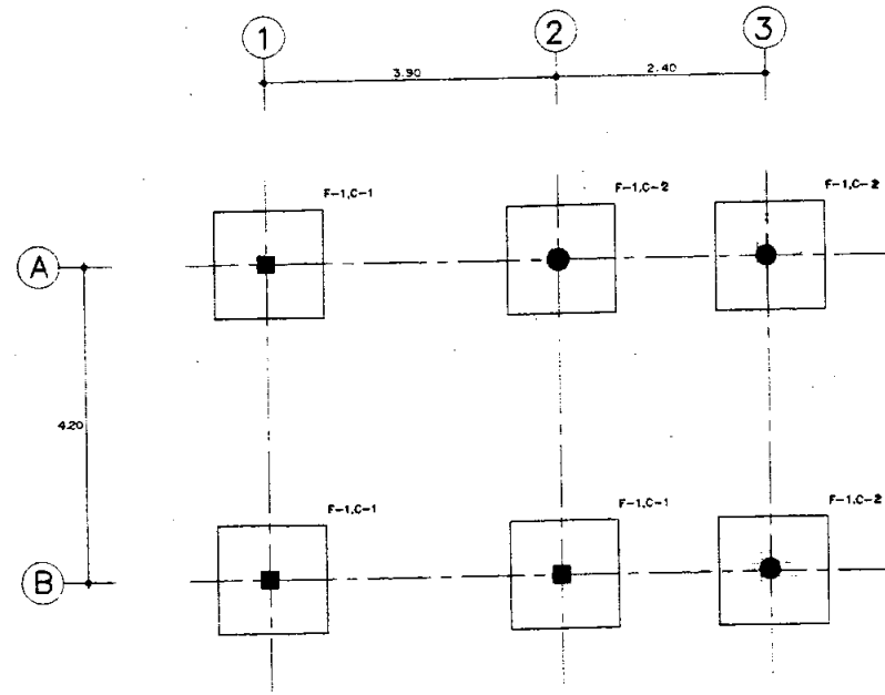
แปลนฐานราก ขนาดส่วน 1 : 50
