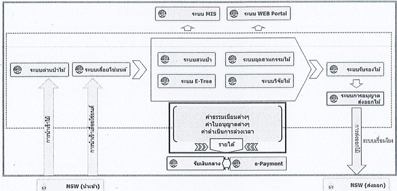
ภาพที่ ๑๑.๑ แผนภาพแสดงการพัฒนาระบบ RFD Single Window กรมป่าไม้
