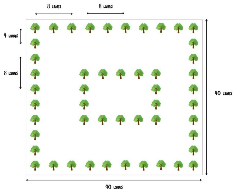
รูปแบบที่ ๒ ปลูกลำไยเศรษฐกิจเป็นแถว ๒ ชั้น ระยะห่างระหว่างต้น ๔ เมตร และระยะห่างระหว่างแถว ๘ เมตร
