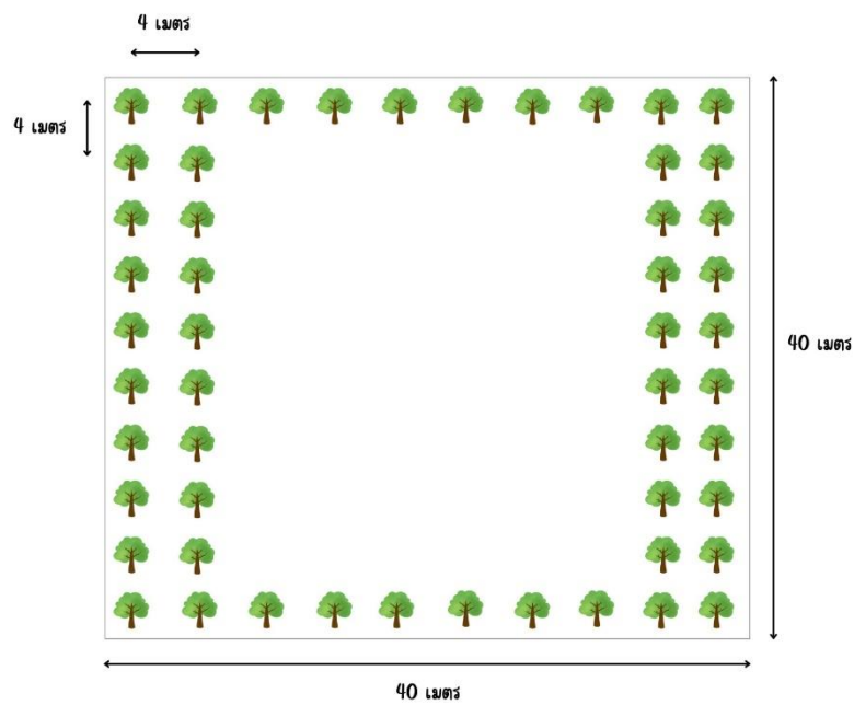
รูปแบบที่ ๓ ปลูกลำไยเศรษฐกิจด้านข้าง ๒ ชั้น ระยะปลูก ๔ x ๔ เมตร
