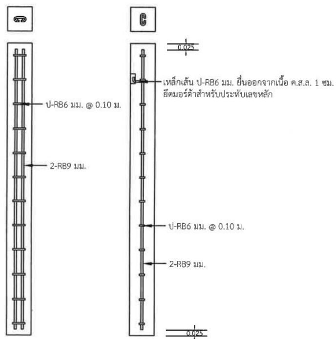
รูปตัดด้านหน้า
