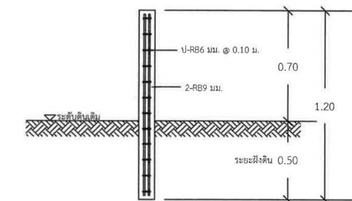
รูปตัด มาตราส่วน 1 : 20
