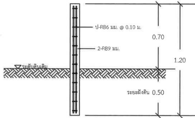
รูปตัด มาตราส่วน 1 : 20
