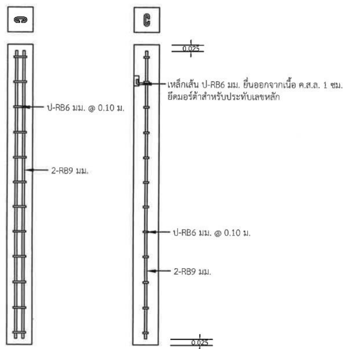
รูปตัดหลักเขตป่าชุมชน
