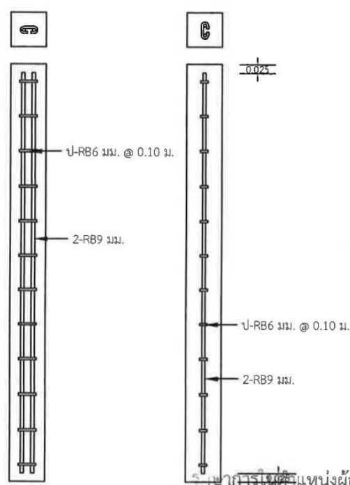
รูปตัดหลักเขตบริเวณเพื่อการใช้ประโยชน์
