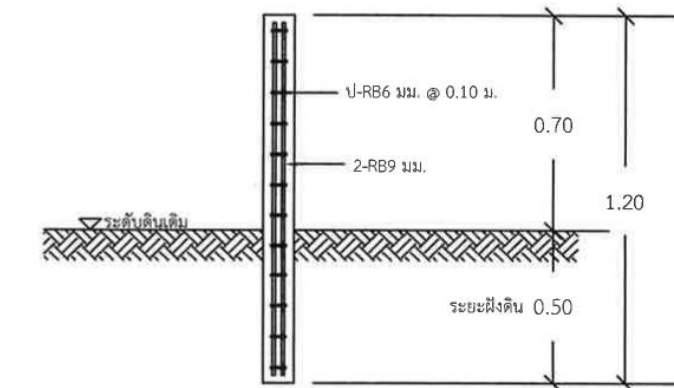
รูปตัด มาตราส่วน 1 : 20
